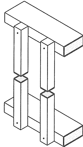
AXONOMETRIC
